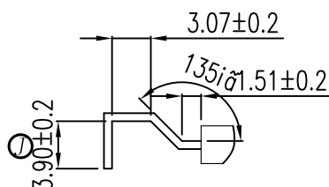
C (2:1) 7PIN脚
