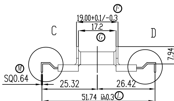
C (2:1) 7PIN脚
