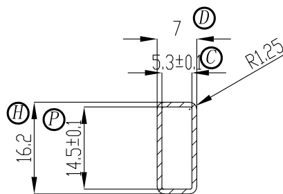
A-A (1 : 1)
